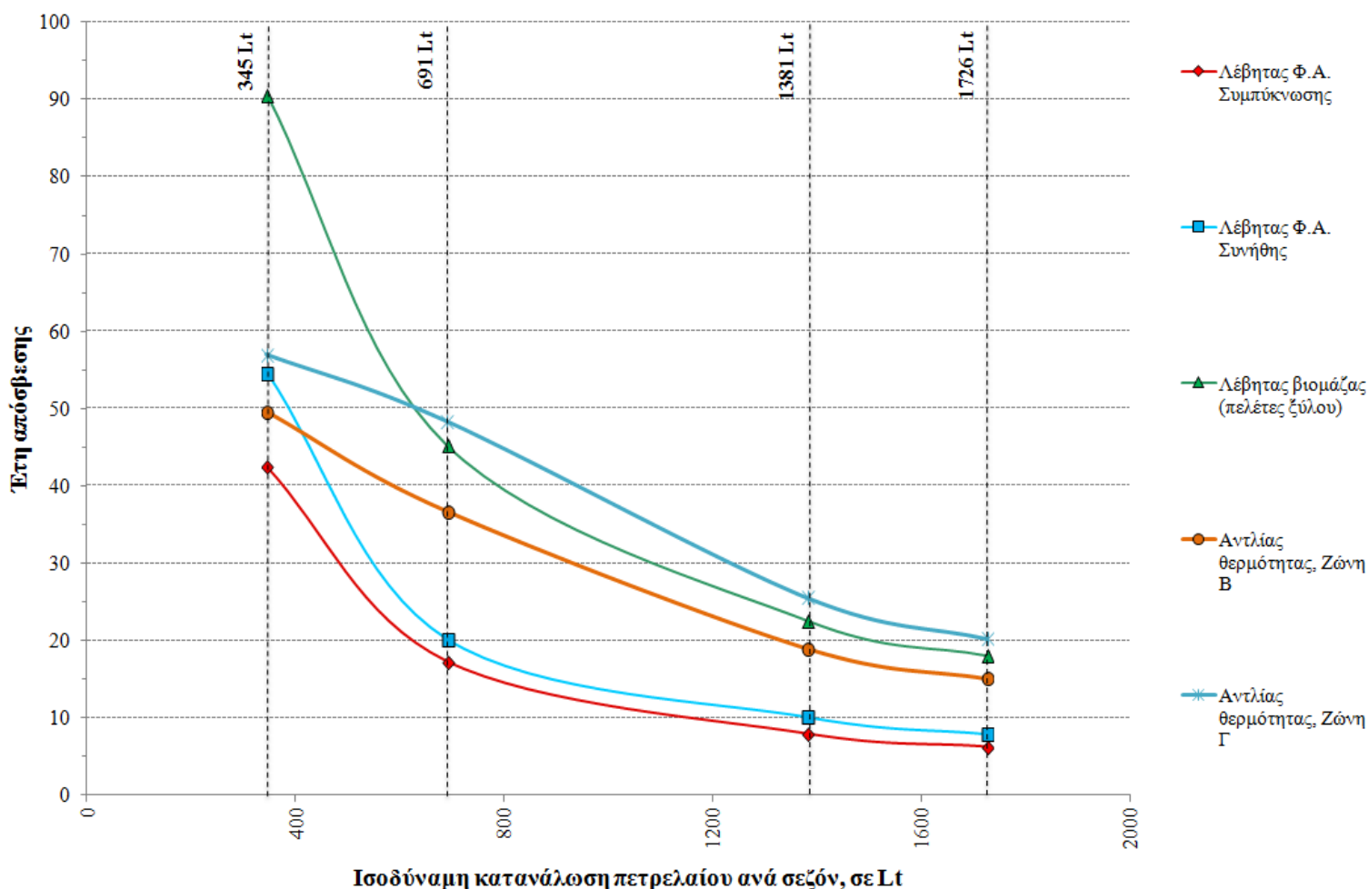
Διάγραμμα 3: Έτη απόσβεσης ανά είδος θερμικού συγκροτήματος για εγκατεστημένη ωφέλιμη θερμική ισχύ 20kW, σε υφιστάμενη εγκατάσταση
