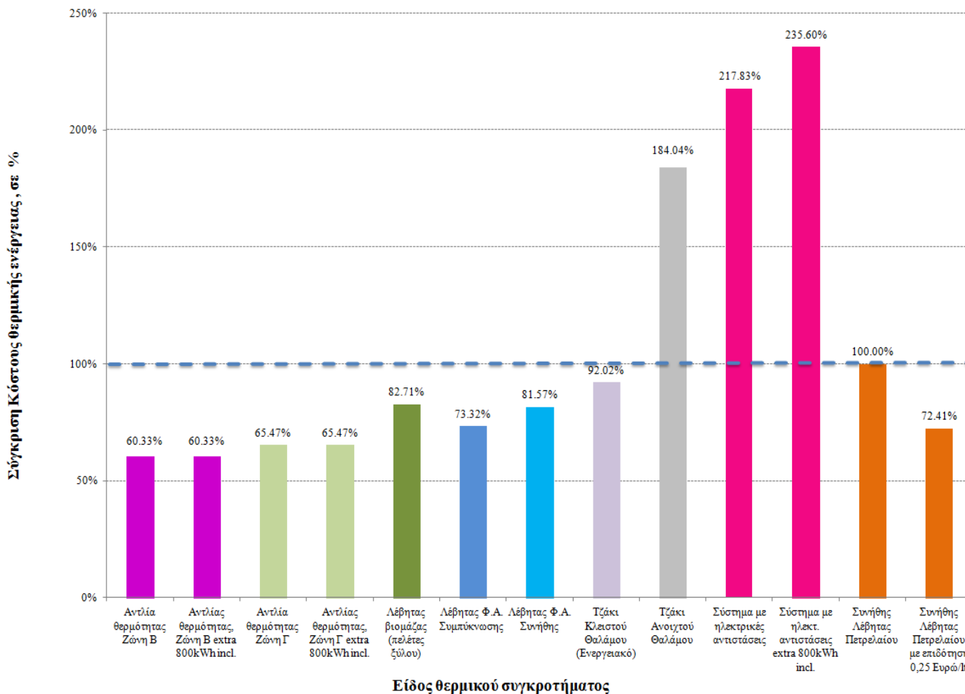
Διάγραμμα 2: Σύγκριση κόστους θερμικής ενέργειας σε %, σε σχέση με το κόστος ενός συγκροτήματος συνήθη λέβητα – καυστήρα πετρελαίου (για τιμή πετρελαίου ~0.906 €/lt), ανά είδος θερμικού συγκροτήματος
